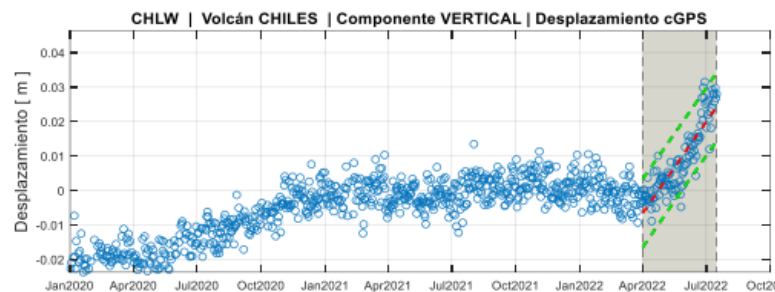
Figura: Serie temporal de datos de desplazamientos (deformación) registrados en dirección vertical por la base cGPS CHLW, ubicada en el flanco SW del volcán Chiles, entre enero de 2020 y julio de 2022. La línea segmentada en color rojo representa la tendencia de los datos desde abril 2022 y las líneas en color verde representan los márgenes de confiabilidad del modelo matemático que la describe.
