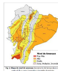
Fig. 1. Mapa de nivel de amenaza. Incremento de temperatura de noche al día y zonas favorables a incendios forestales.
