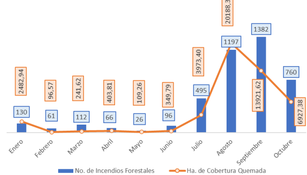
Recurrencia de eventos vs. Ha. de coberturas vegetal quemada por mes
