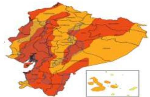
Estimación de Máxima Precipitación Acumulada Diaria
