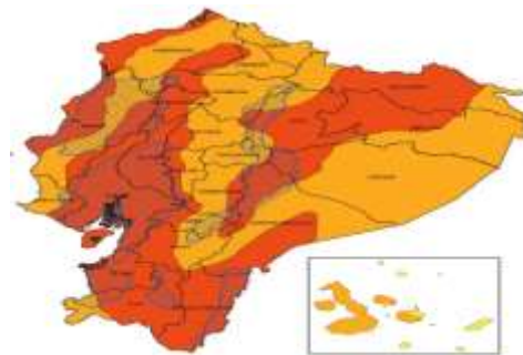
Estimación de Máxima Precipitación Acumulada Diaria
